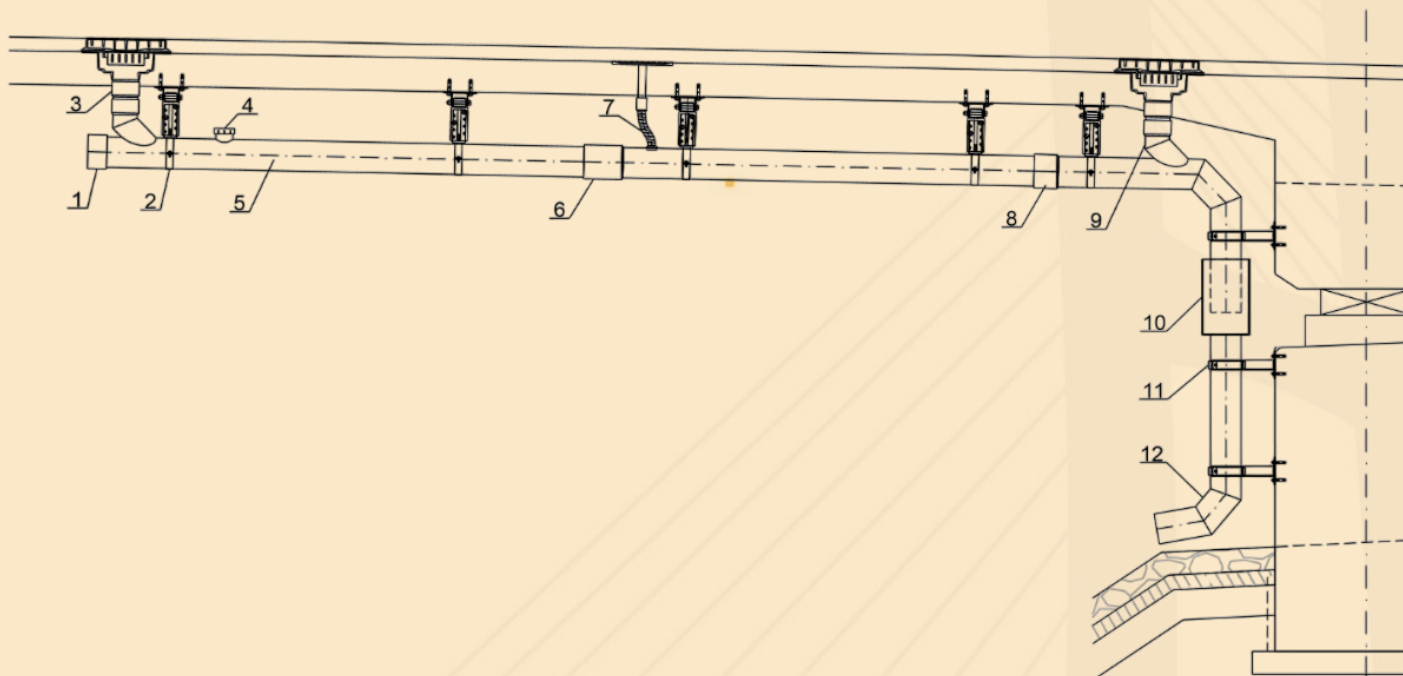
Obrázok 1: Schéma zostavy odvodnenia KOGA Bau
